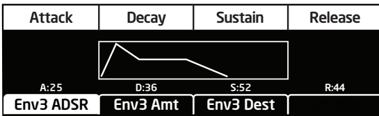
TAB 1 - Env ADSR
